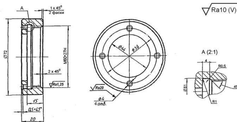
Деталь - ШТУЦЕР
