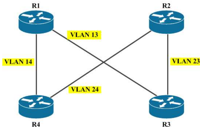
Рисунок 3 - Логическая топология №2
