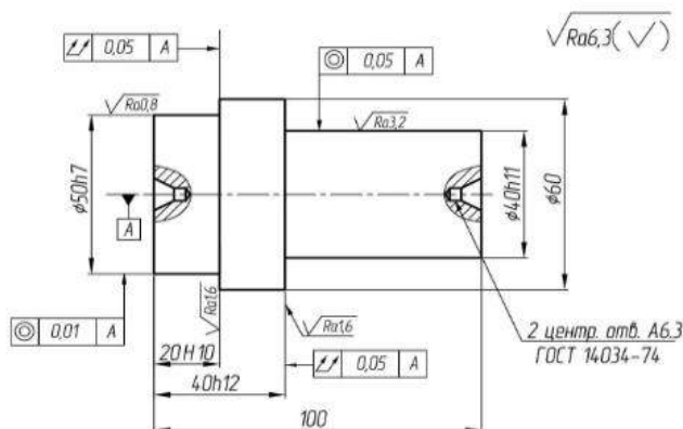
Рисунок – Эскиз детали «вал»
