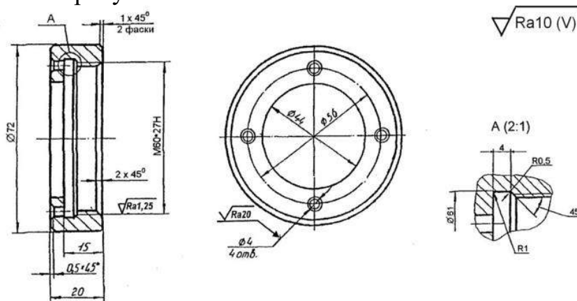
Деталь - ГАЙКА НАКИДНАЯ
