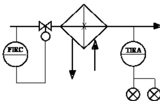
Рис.№4 Упрощенная функциональная схема автоматизации
