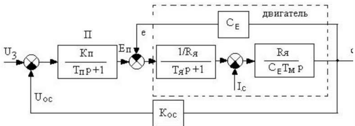
Структурная схема САР
