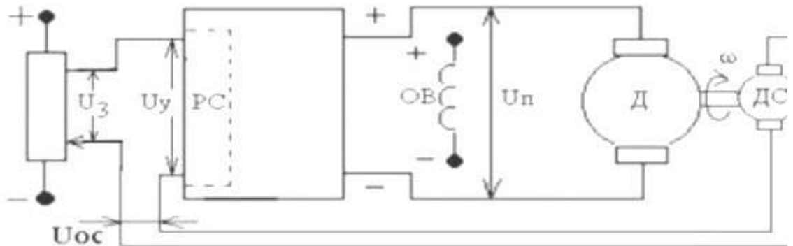
САР двигателя постоянного тока с обратной связью по скорости
