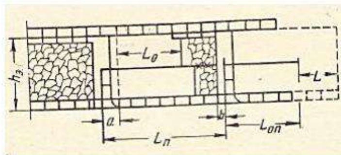
Графическая модель №2 - длинные столбы с доставкой угля к заднему бремсбергу
