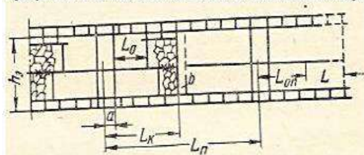
Графическая модель №3 - длинные столбы с двусторонними бремсбергами
