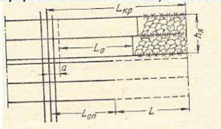
Графическая модель №1 - - спаренные столбы при панельной подготовке;
