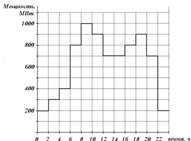
Рис. ПЗ. Прогнозный суточный график нагрузки энергосистемы
