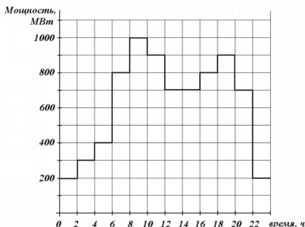
Рис. ПЗ. Прогнозный суточный график нагрузки энергосистемы
