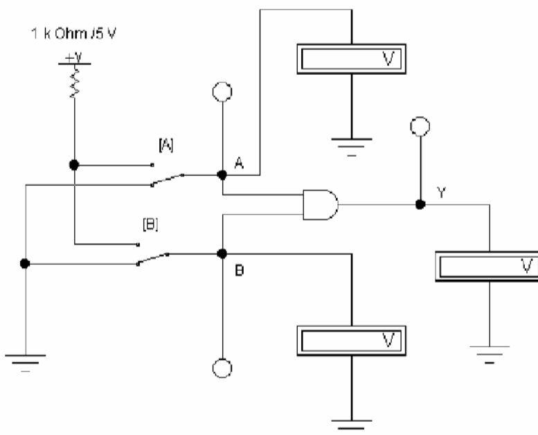
Рис. 1. – Логическая функция «И»
