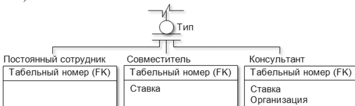
Рис. 4. Иерархия наследования (полная категория)
