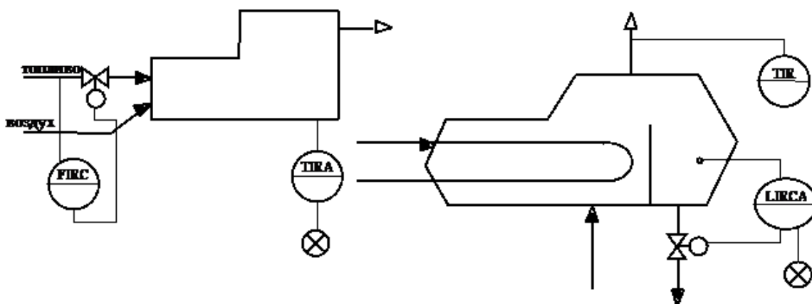
Рис.№6 Упрощенная функциональная схема автоматизации
