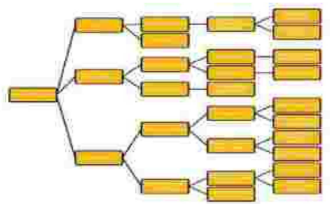
Рисунок 1. «Дерево» целей.
