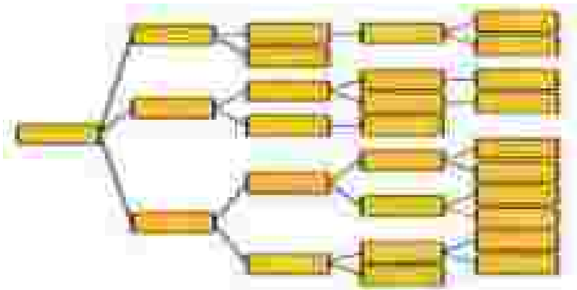
Рисунок 1. «Дерево» целей.
