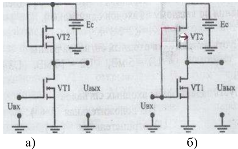
Рис. 1. Схемы логических элементов к заданиям 1, 2
